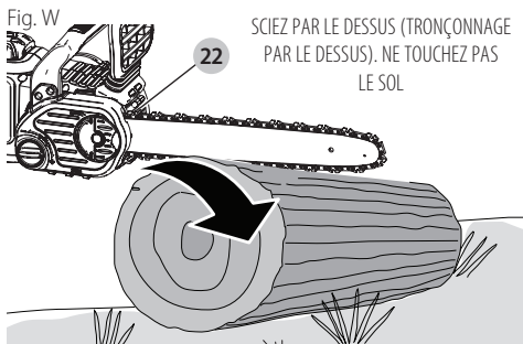
Figure X- Si la pièce à scier est soutenue par une extrémité, sciez d'abord 1/3 du diamètre par le dessous (tronçonnage par le dessous). Finalisez ensuite la coupe en sciant par le dessus pour rejoindre la première ligne de coupe.
